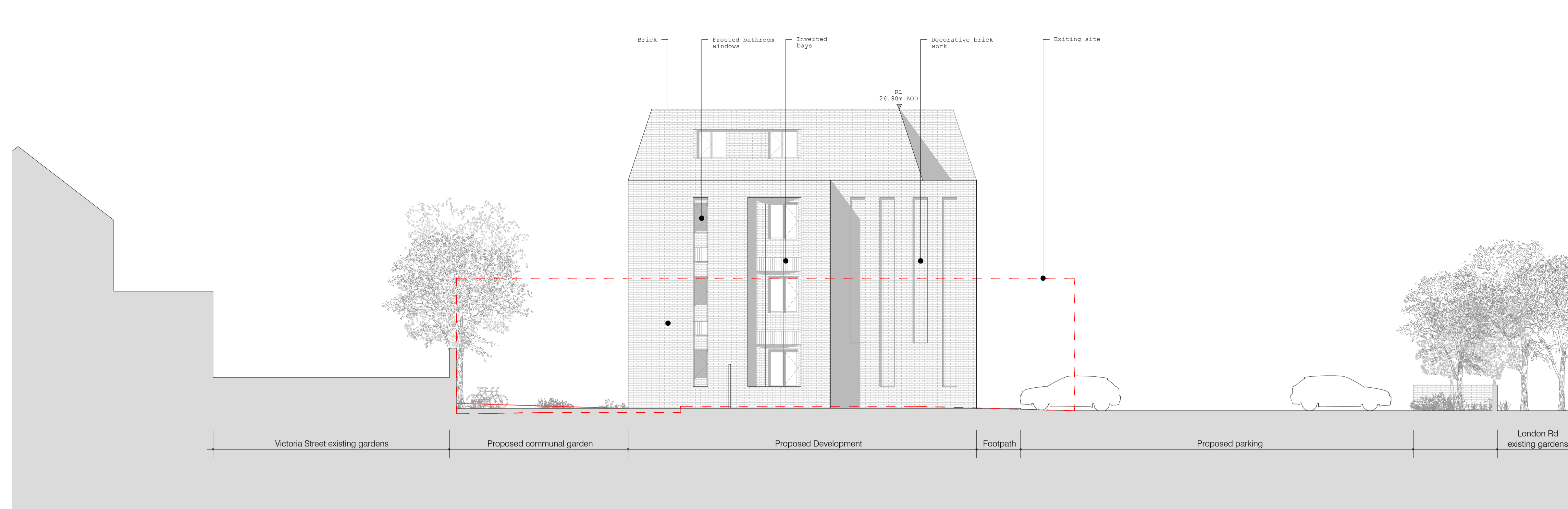
Elevation C-C'
