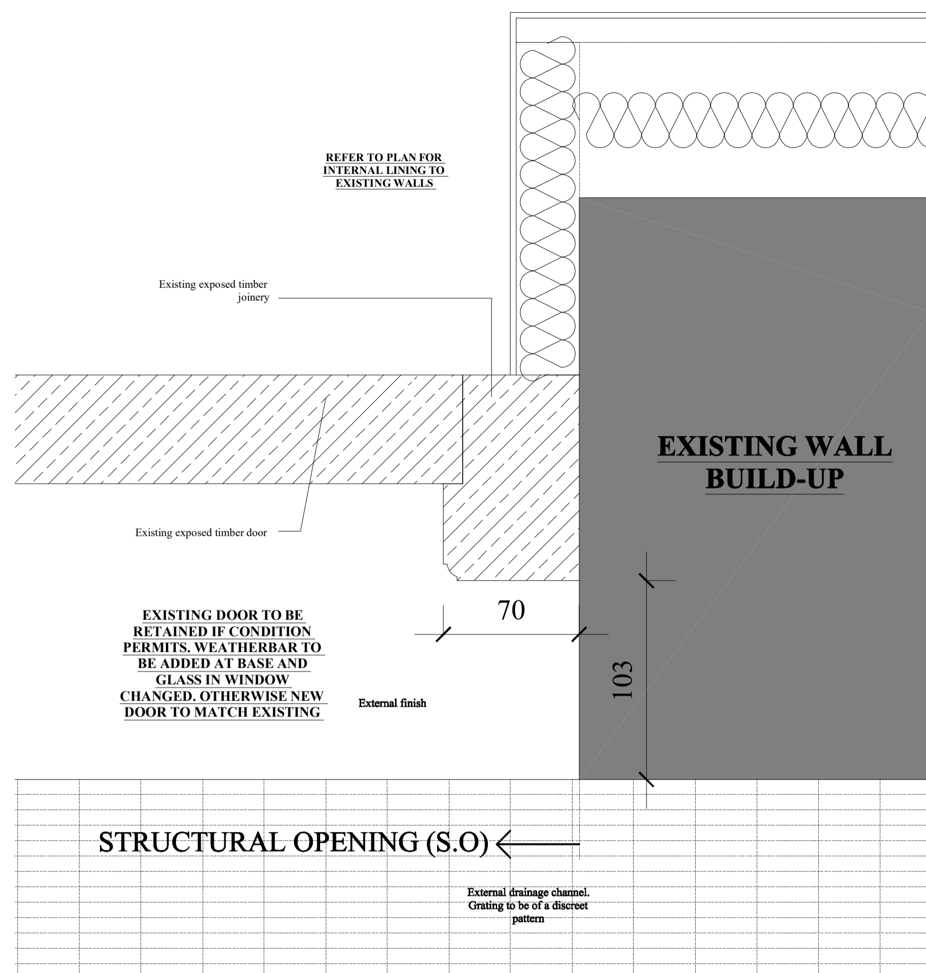
GF-D-01 JAMB PLAN DETAIL
